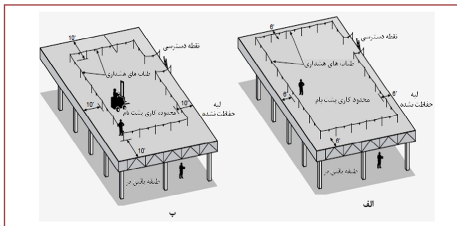
شکل ۴۸- سیستم طناب هشدار بدون استفاده از وسایل متحرک (الف) و با استفاده از وسایل متحرک (ب)
